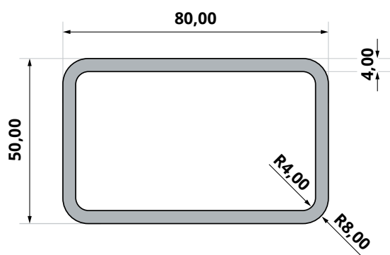
Koud vervaardigd Stalen koker
