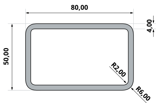
Blank-gelaste en RVS koker
